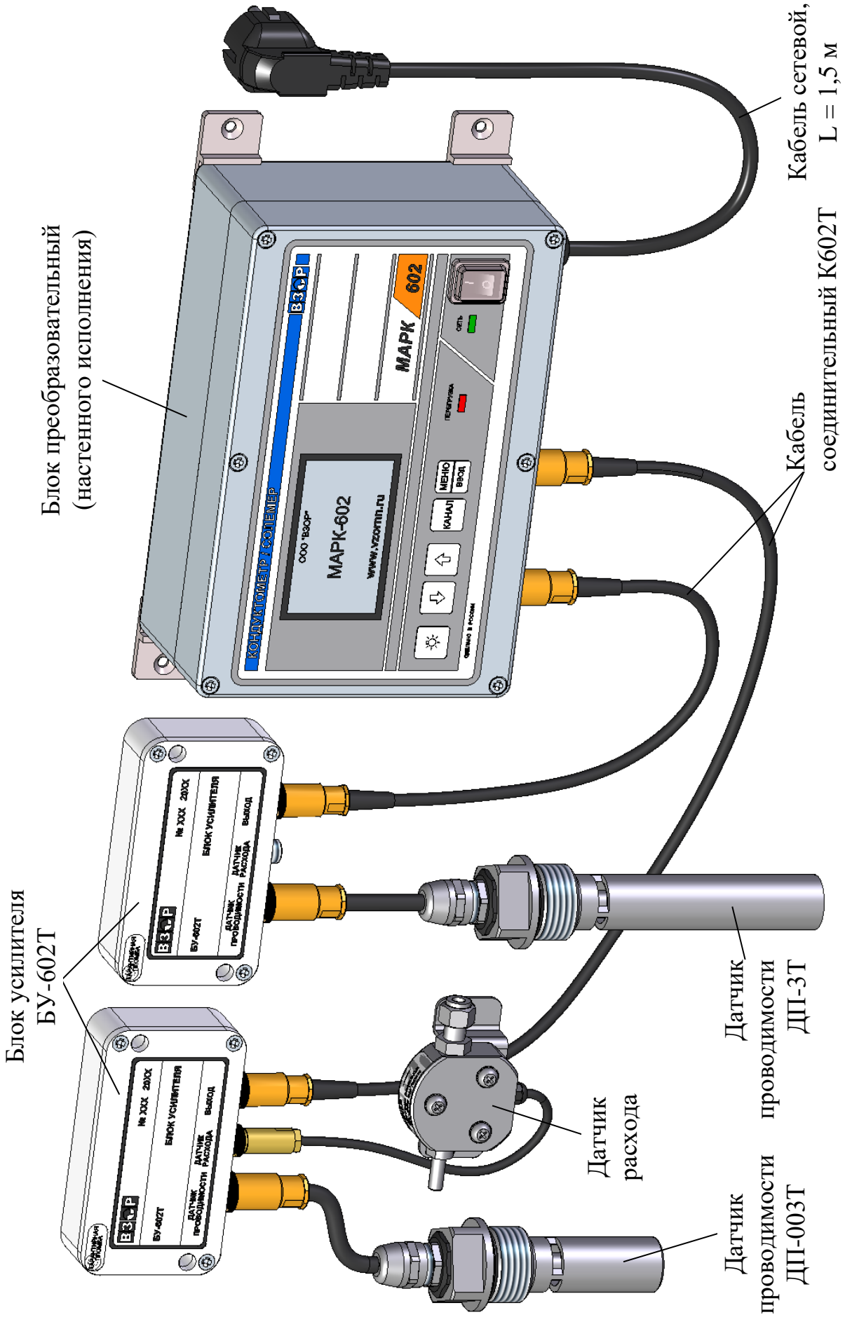
Рисунок 1.1 – Кондуктометр-солемер МАРК-602Т/1
