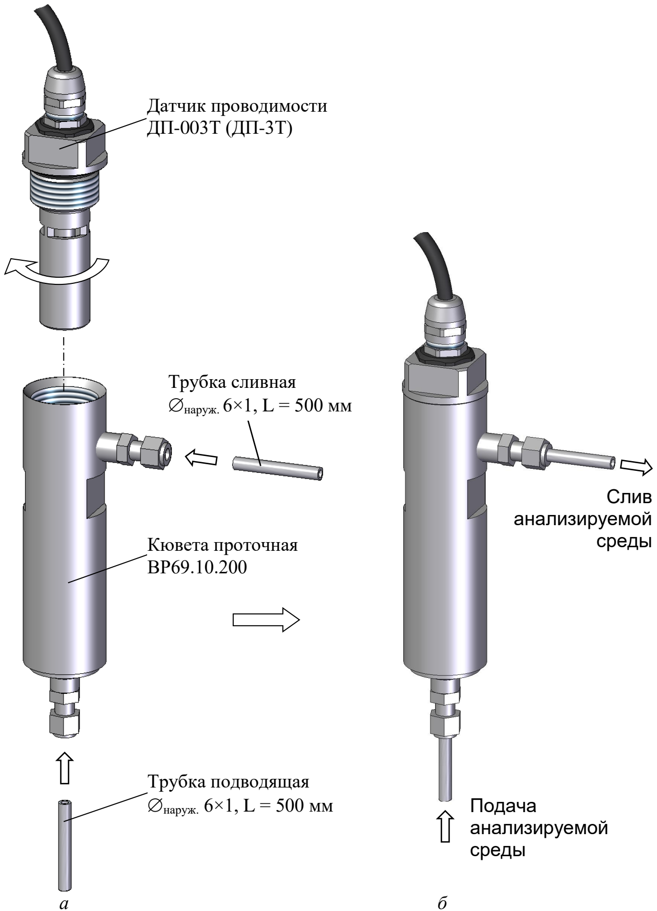
Рисунок 2.11 – Расположение датчика проводимости ДП-003Т в кювете проточной ВР69.10.200 при проточном способе измерений
