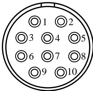
Вилка РСГ10ТВ
