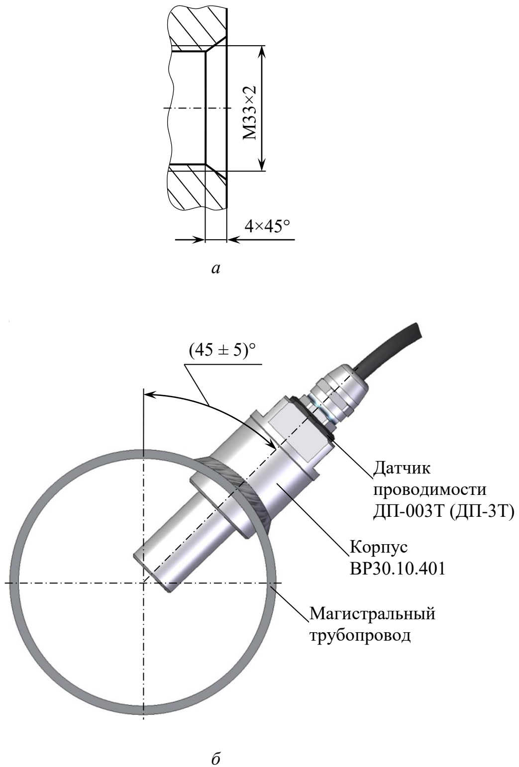
Рисунок 2.13 – Расположение датчика проводимости ДП-003Т (ДП-3Т) в магистральном трубопроводе
