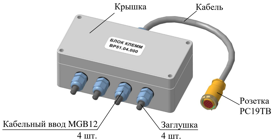
Рисунок 2.6 – Блок клемм VP51.04.000
