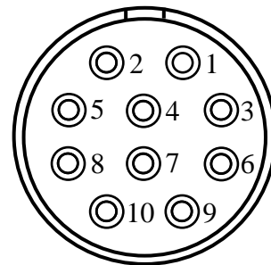
Розетка РС10ТВ
