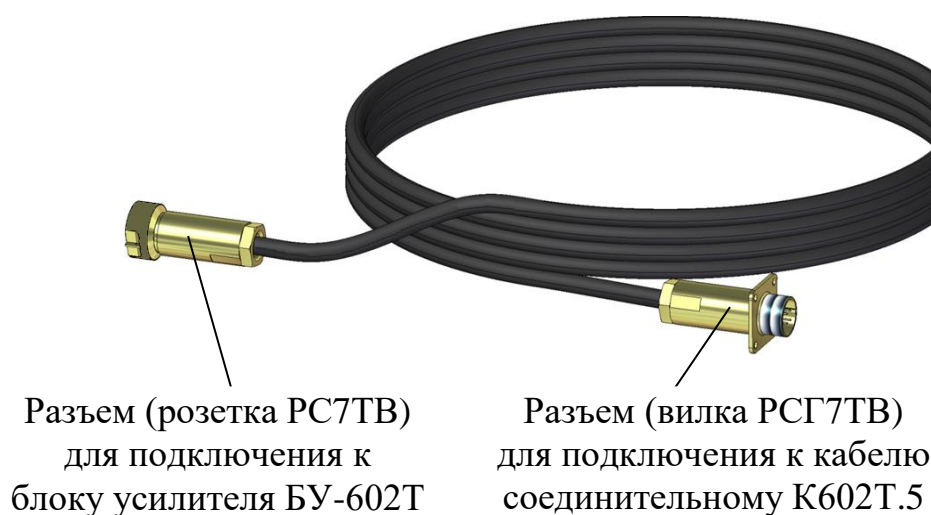
Рисунок 2.8 – Вставка кабельная ВК602Т.Л ВР69.05.000
