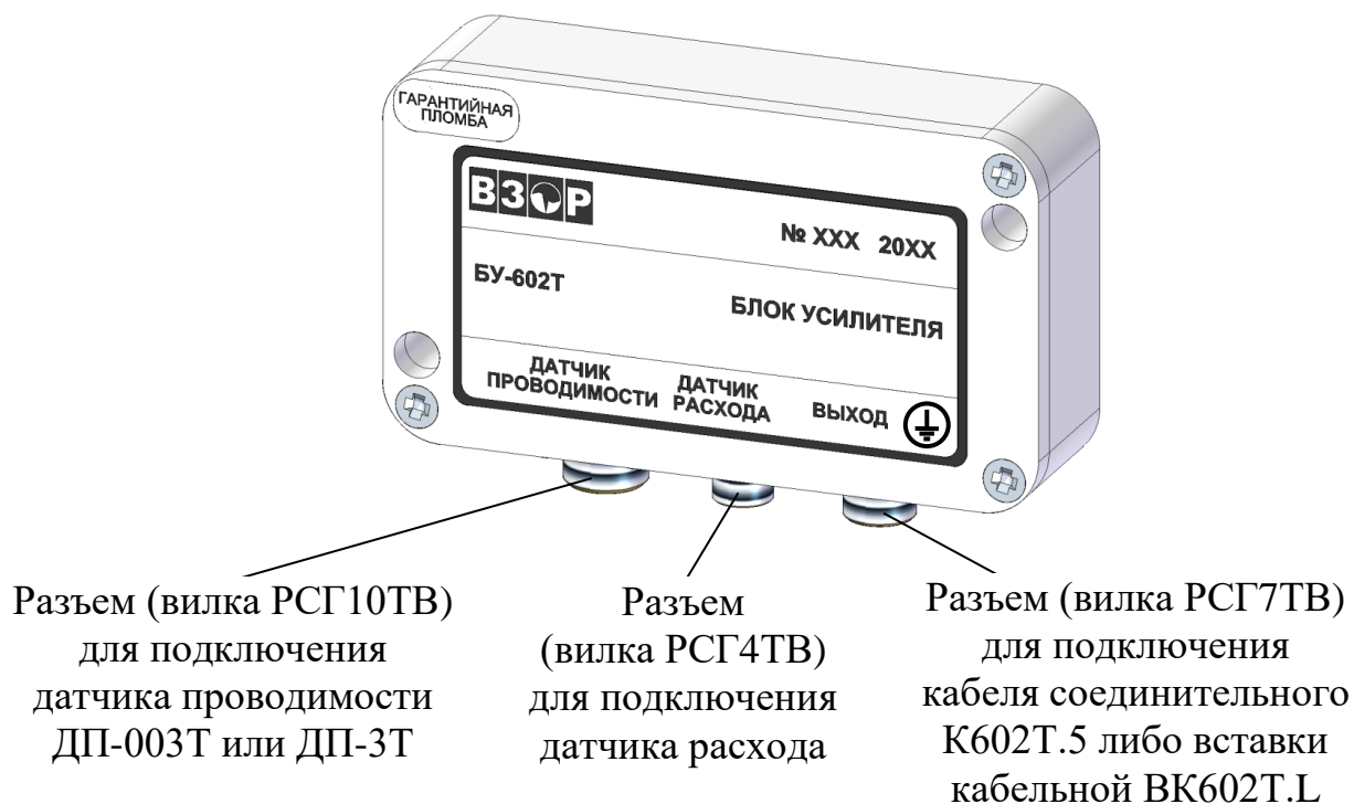
Рисунок 1.5 – Блок усилителя БУ-602Т
