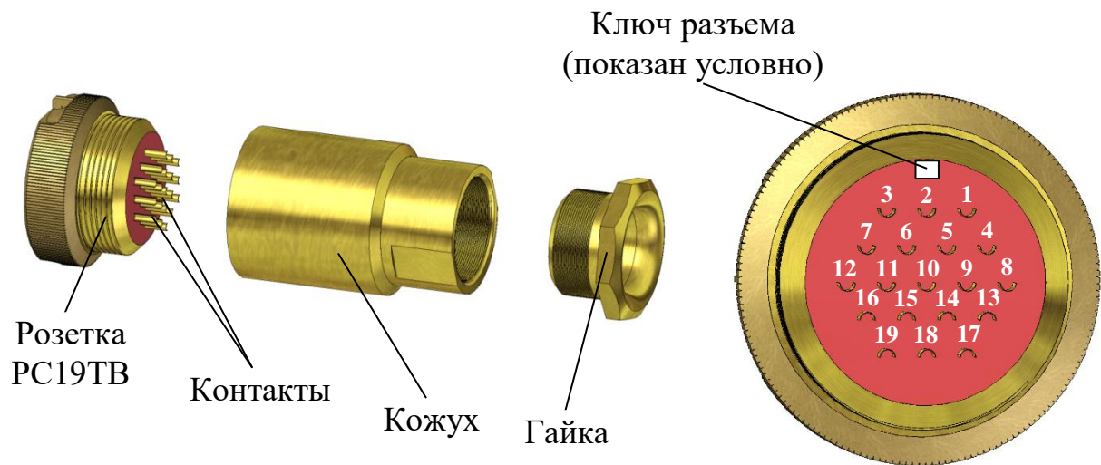
а – Конструкция розетки
