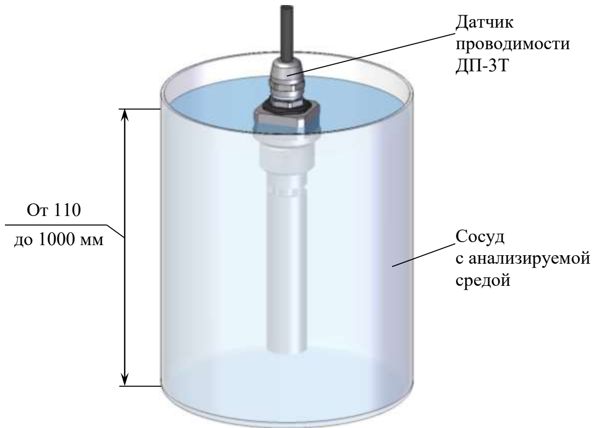
Рисунок 2.9 – Пример расположения датчика проводимости в сосуде с анализируемой средой при погружном способе измерений
