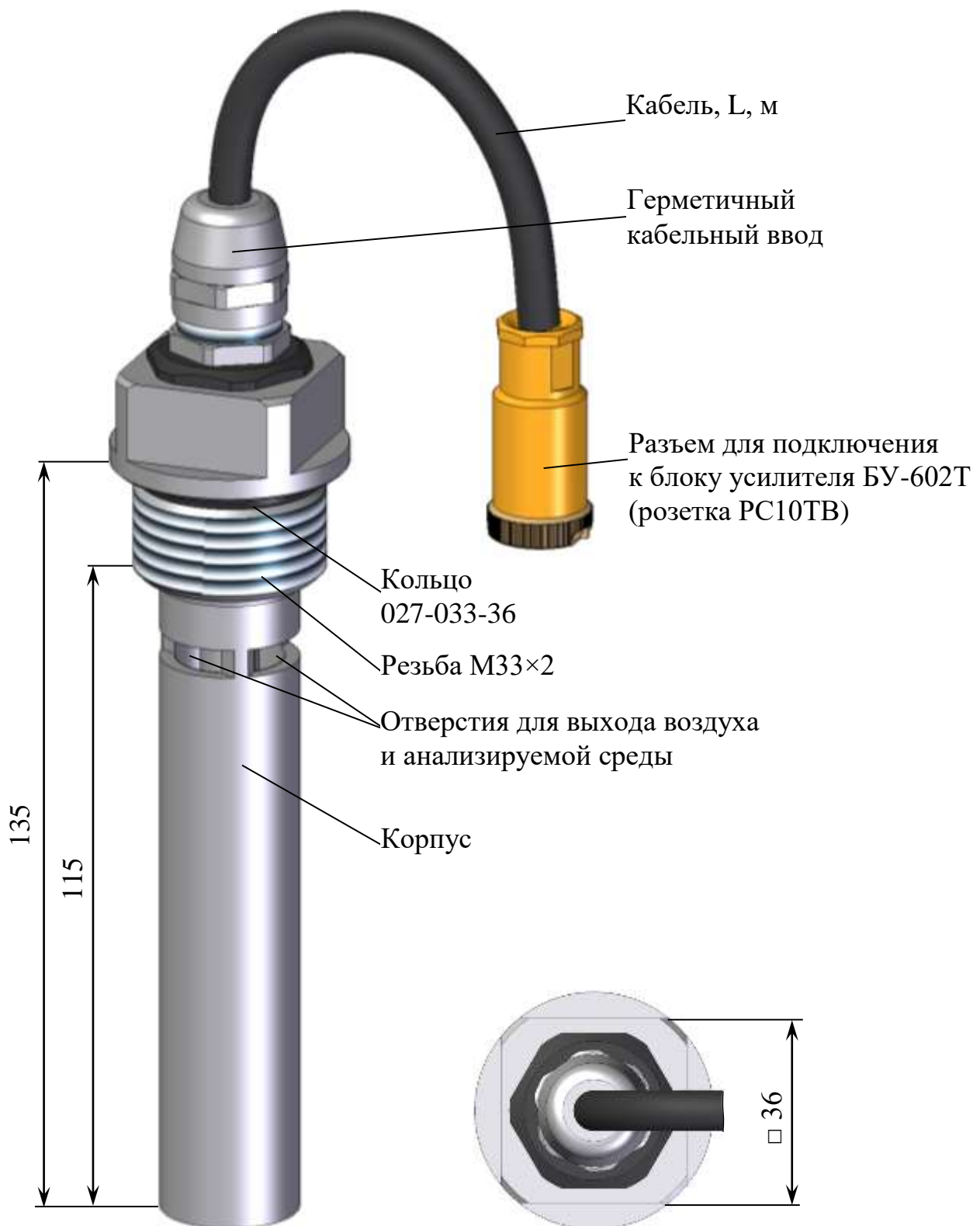
Рисунок 1.7 – Датчик проводимости ДП-3Т
