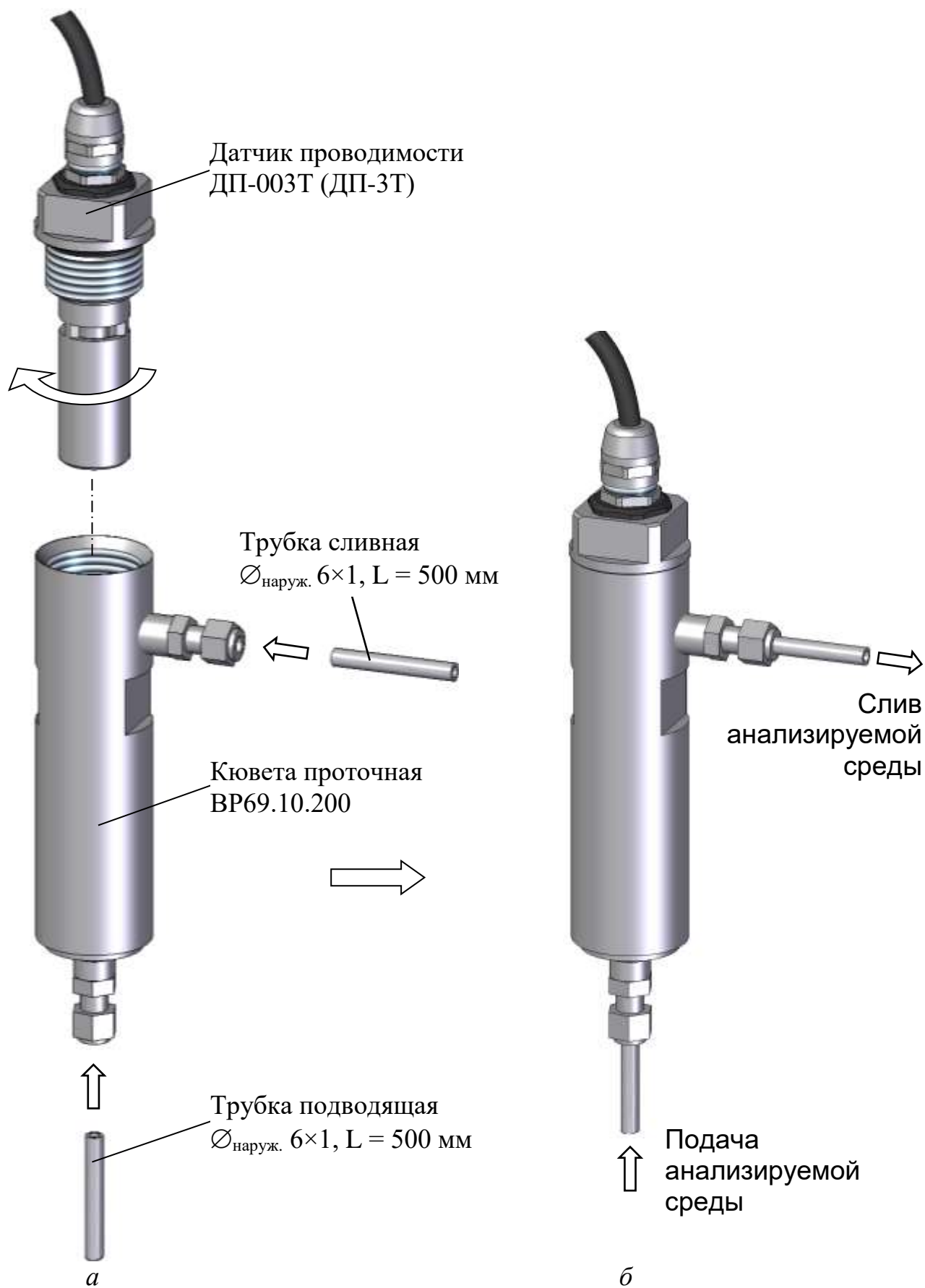
Рисунок 2.11 – Расположение датчика проводимости ДП-003Т в кювете проточной VR69.10.200 при проточном способе измерений
