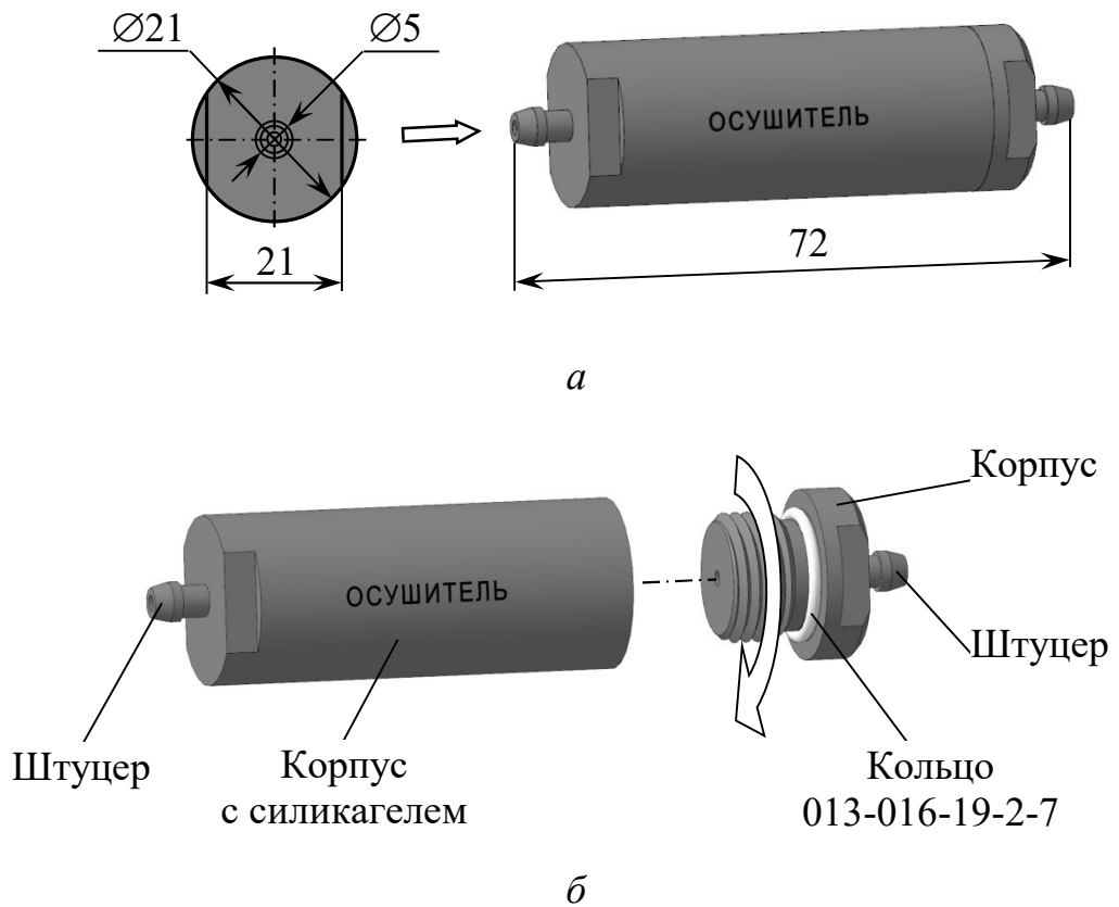
Рисунок 1.4 – Осушитель ВР84.04.120
