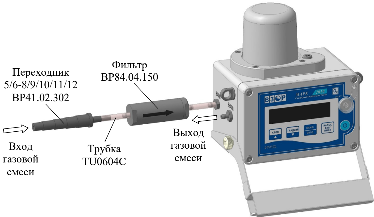
Рисунок 2.11 – Проведение измерений
